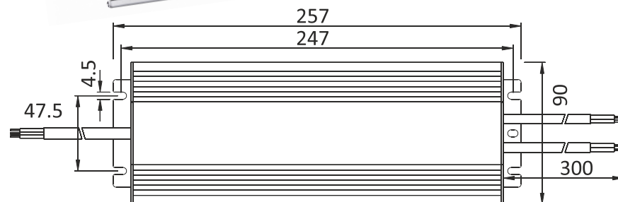
WYMIARY
